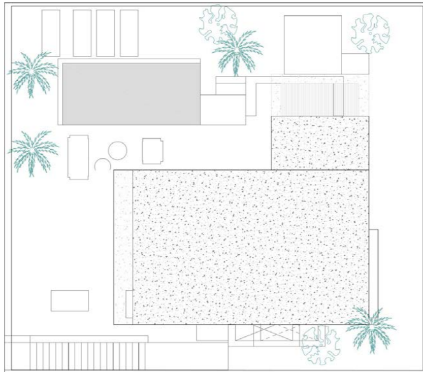
Planta cubierta
