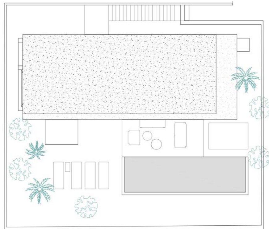
Planta cubierta
