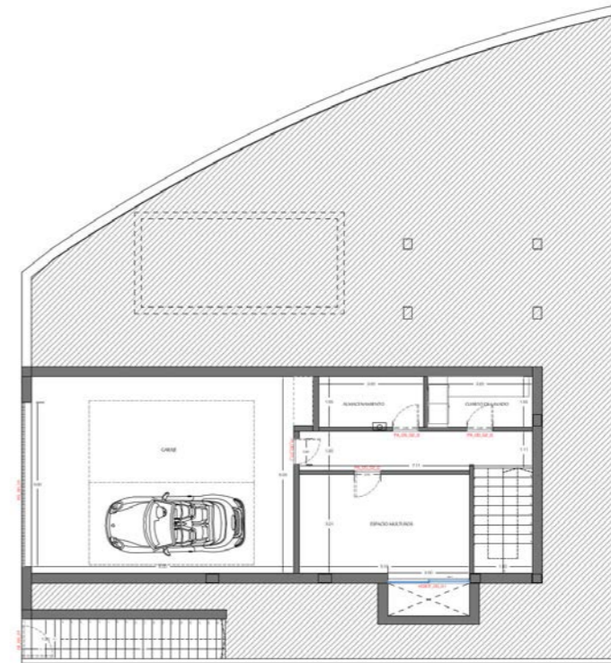
Planta sótano
